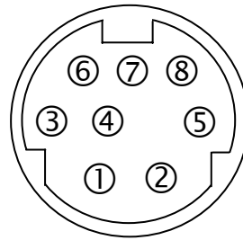
8PIN Mini Din 公座 (线缆接头上视图)
