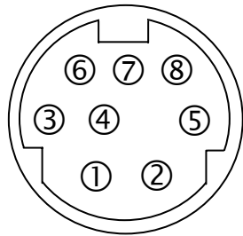
8PIN Mini Din 公座 (线缆接头上视图)
