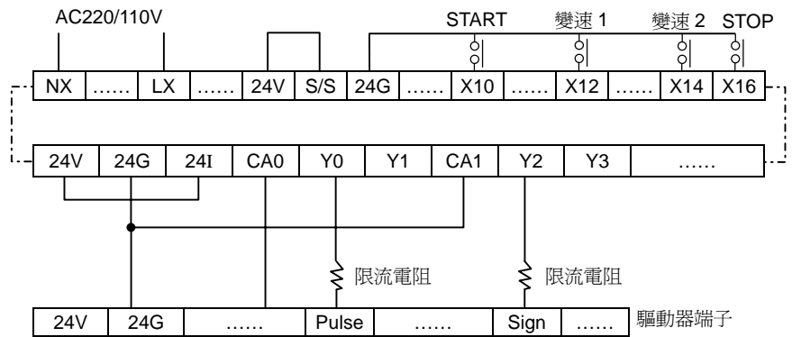
◆接線圖
